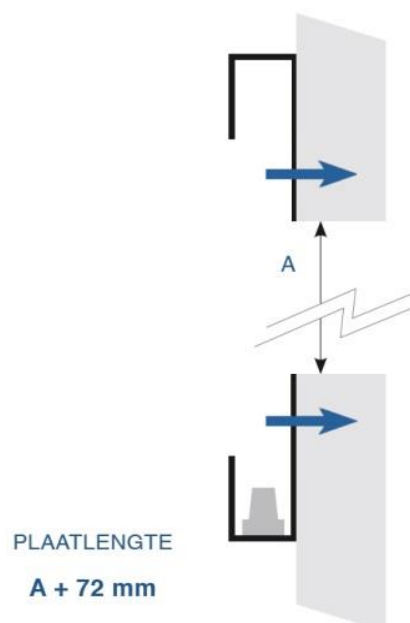
Figuur 2 Monteren voor het raamwerk
