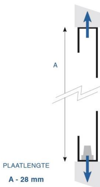
Figuur 1 Monteren in het raamwerk
