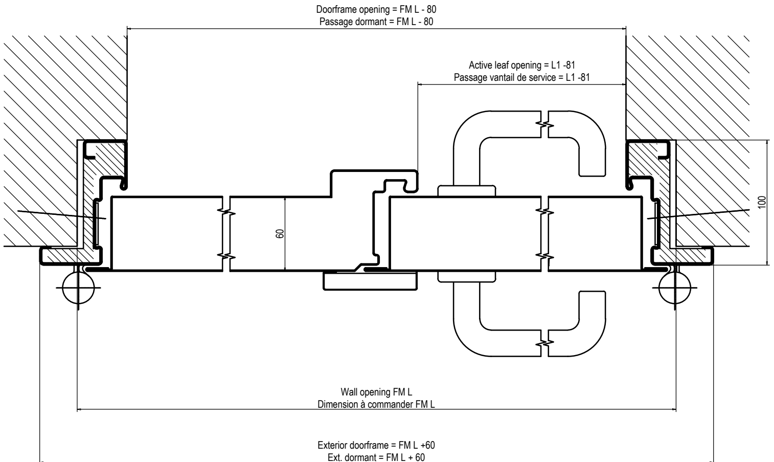
Horizontal cross section Coupe horizontale
