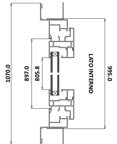
SEZIONE BB
