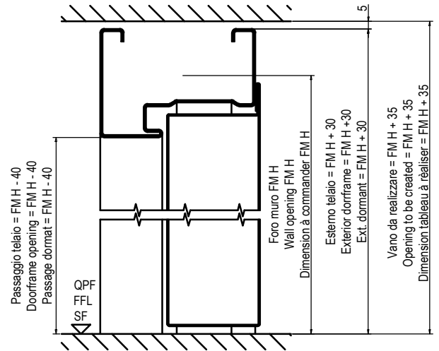
Sezione verticale Vertical cross section Coupe vertical
