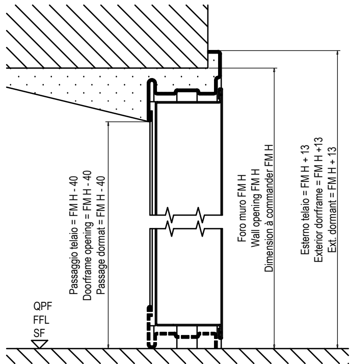
Sezione verticale Vertical cross section Coupe vertical
