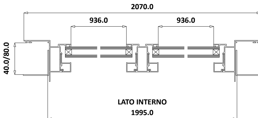
Aanzicht A-A
