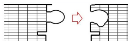
Detail van het Kliksysteem
