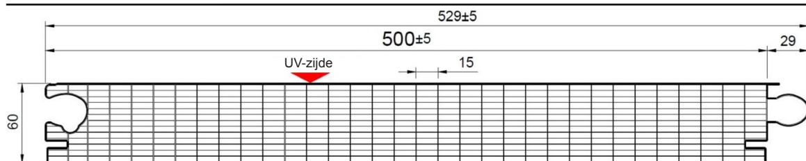
Doorsnede
